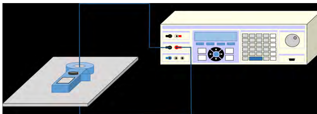
Figura 1. Circuito de medición de una espira para calibración de pinza amperimétrica
