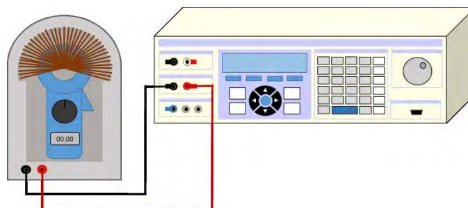
Figura 2. Comparación indirecta pinza amperimétrica y calibrador patrón con bobina 50 vueltas
